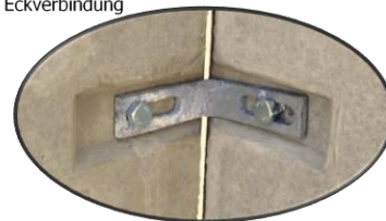
Detail 1 Eckverbindung
