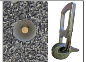
Detail hijshaak
