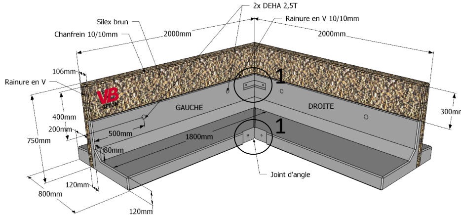
Détail pied
