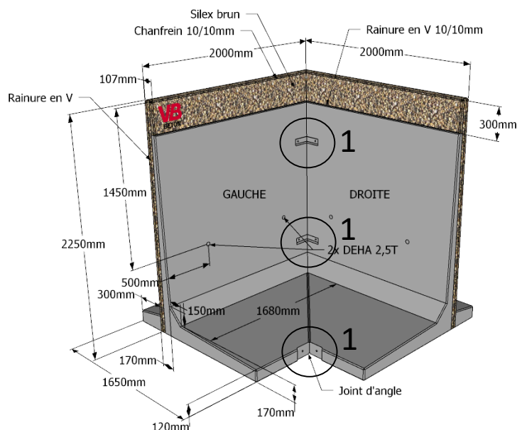
Détail 1. Joint d'angle
